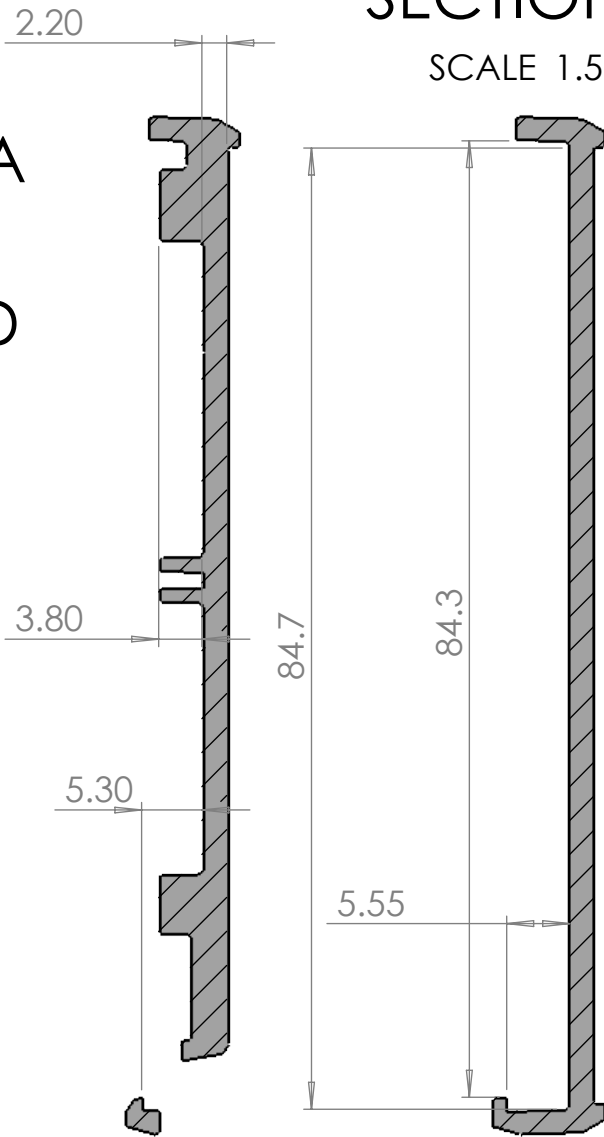
SECTION J-J SCALE 1.5 : 1
